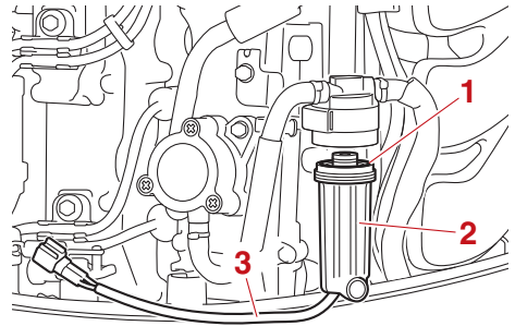
1. Junta tórica 2. Taza del filtro 3. Cable del interruptor de detección de agua
