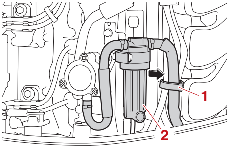
1. Soporte 2. Filtro de gasolina
