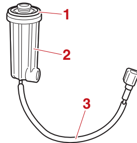
1. Junta tórica 2. Taza del filtro 3. Cable del interruptor de detección de agua
