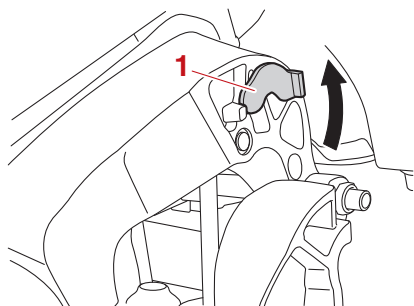
1. Soporte del motor elevado
