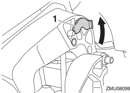
1. Ankip-Arretierungshebel
