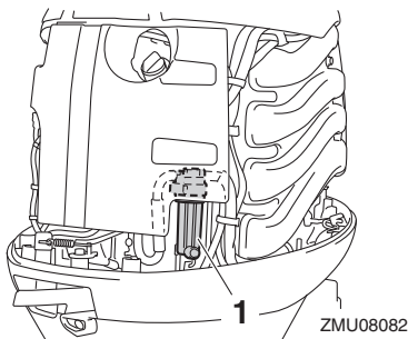
1. Kraftstofffilter
