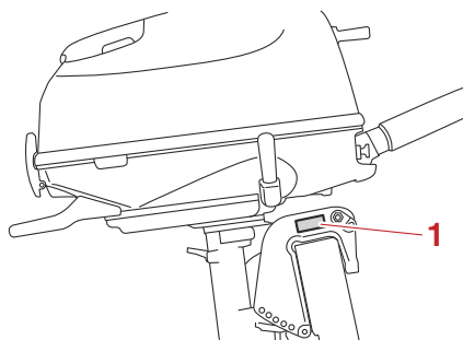
1. Emplacement du marquage CE
