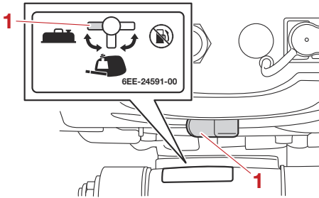
1. Position du réservoir de carburant portable
