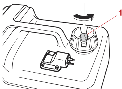
1. Vis de mise à pression atmosphérique
