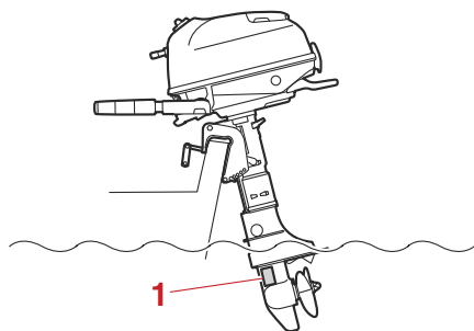
1. Entrée d'eau de refroidissement
