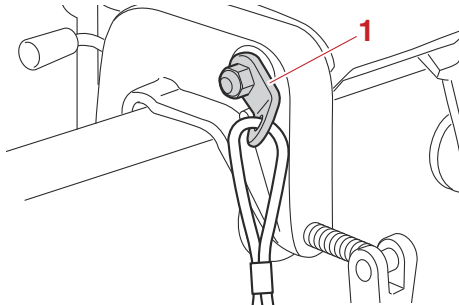
1. Fixation pour câble de sécurité
