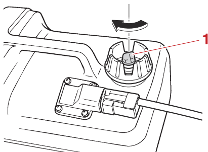
1. Vis de mise à pression atmosphérique
