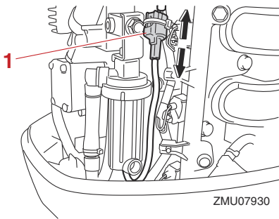
1. Wasseranzeigeschalter-Stecker
