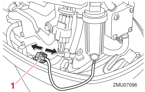
1. Wasseranzeigeschalter-Stecker
