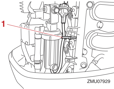
1. Kabelbinder
