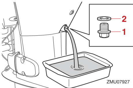
1. Ablassschraube 2. Dichtung
