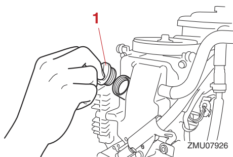
1. Öltankdeckel
