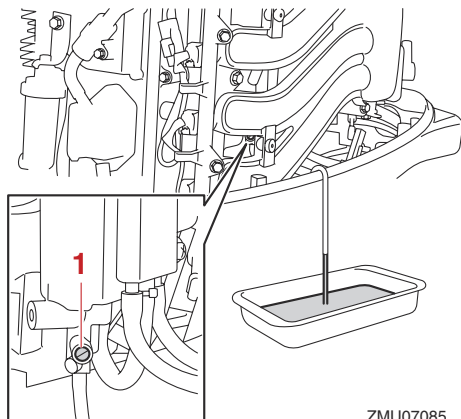
1. Ablassschraube
