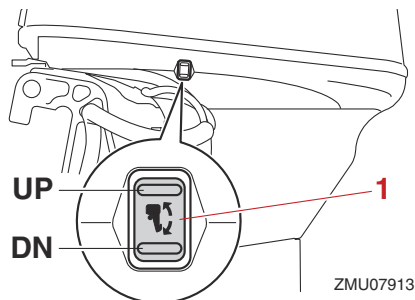
1. PTT-Schalter
