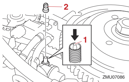
1. Ablassschraube
