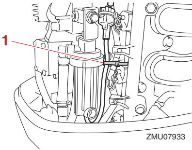
1. Kabelbinder
