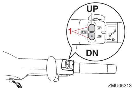
1. Variabler Schlepp-U/min-Schalter
