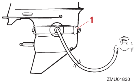
1. Conector de lavado
