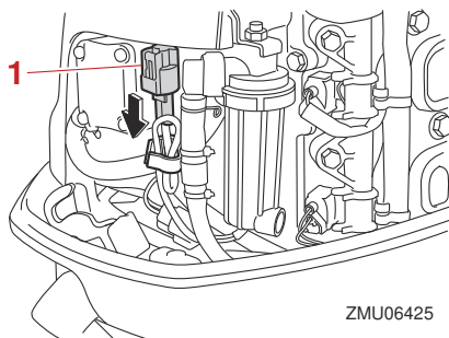
1. Acople del interruptor de detección de agua
