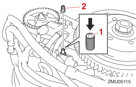
1. Varilla de conexión del estrangulador 2. Tapa
