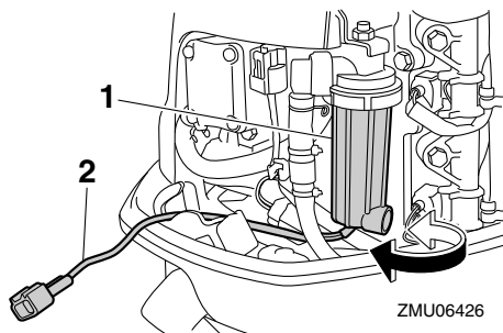
1. Filtergehäuse 2. Wasseranzeigeschalter-Kabel
