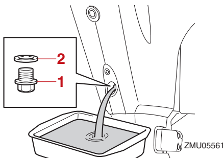
1. Aftapschroef 2. Pakking
