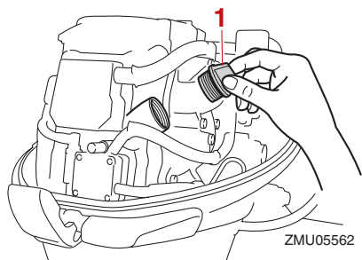
1. Olievuldop
