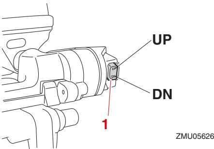
1. Kantelbekrachtigingsschakelaar
