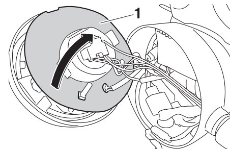
1. Abdeckung
