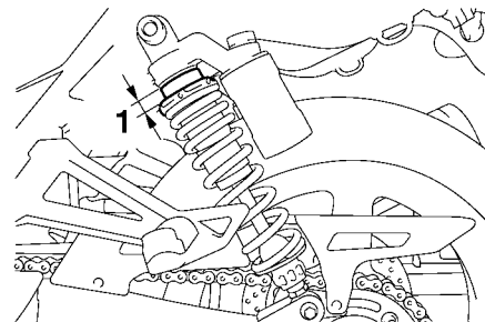
1. Abstand A
