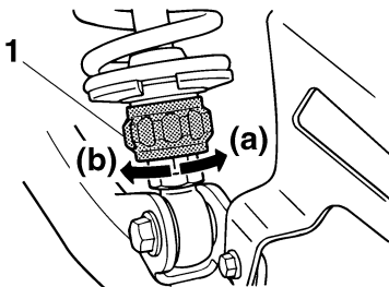
1. Zugstufendämpfungs-Einstellknopf
